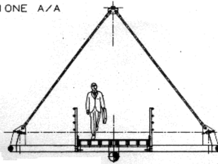
SEZIONE A/A
