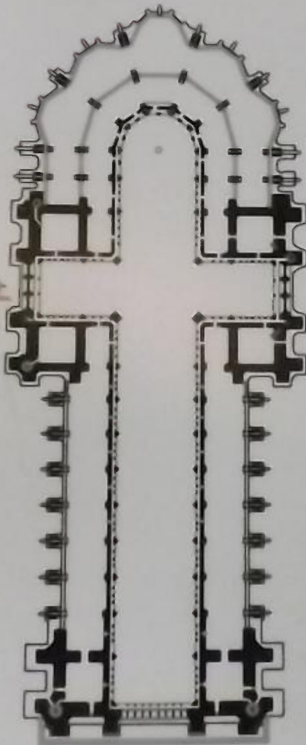
NIVEAU DU TRIFORIUM
