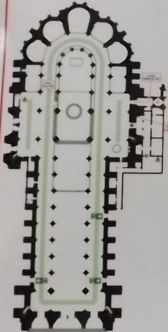
REZ-DE-CHAUSSEE
