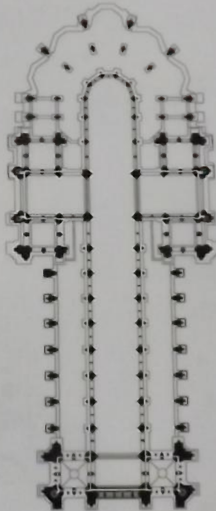
NIVEAU DES FENETRES HAUTES
